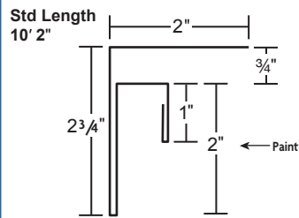
G-Rib F&J
