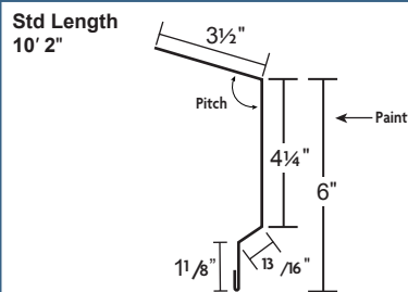
Fascia Trim
